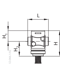
VGU DN 15-25
